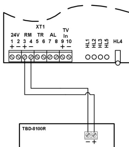
שרטוט 6 חיבור מכלול חיווי אופציונאלי TBD-8100R לגלאי
